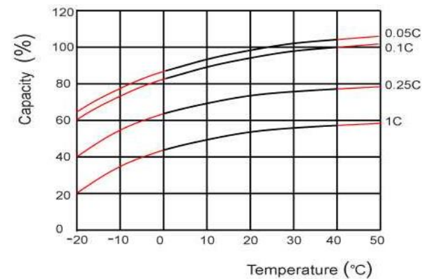
Зависимость емкости от температуры
